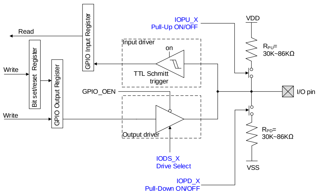
图 6-3 I/O 端口的输出配置
