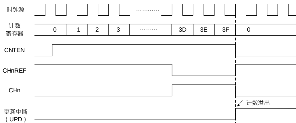
图 20-21 单脉冲模式
