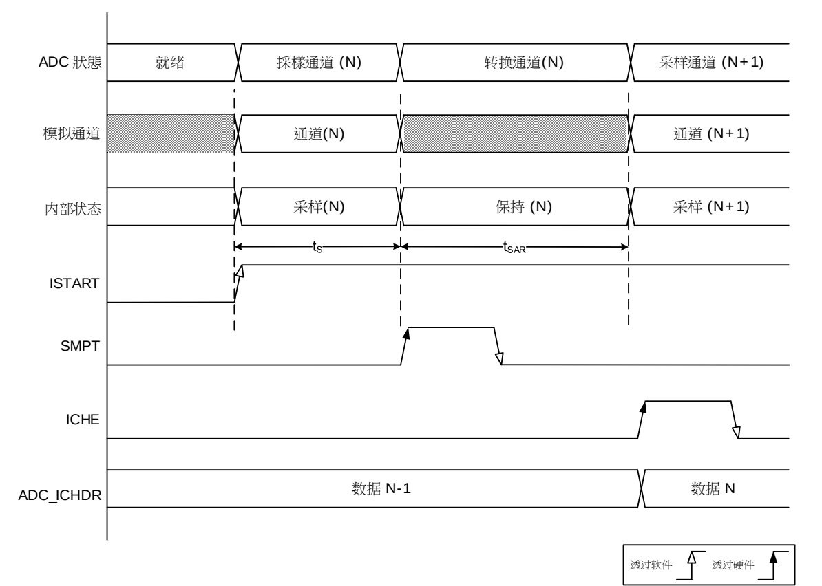
图 16-5 ADC 插入转换
