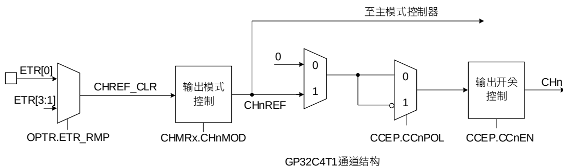
图 19-14 捕获或比较通道的输出部分
