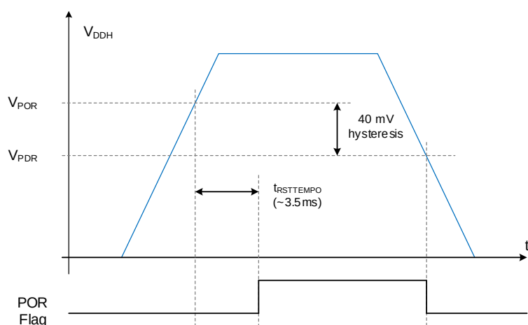
图 3-2 POR/PDR 复位
