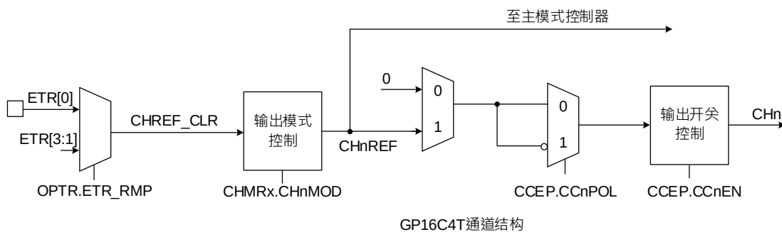
图 20-14 捕获或比较通道的输出部分
