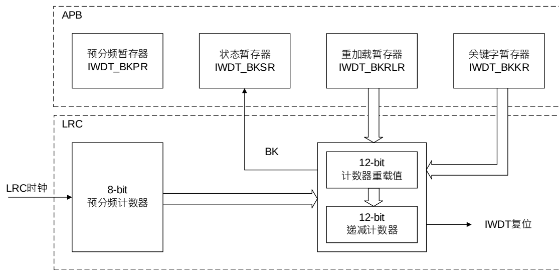
图 23-1IWDG 架构图
