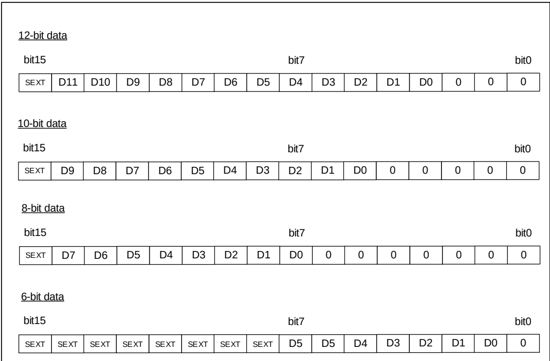
图 16-15 左对齐(使用偏移,有符号值)
