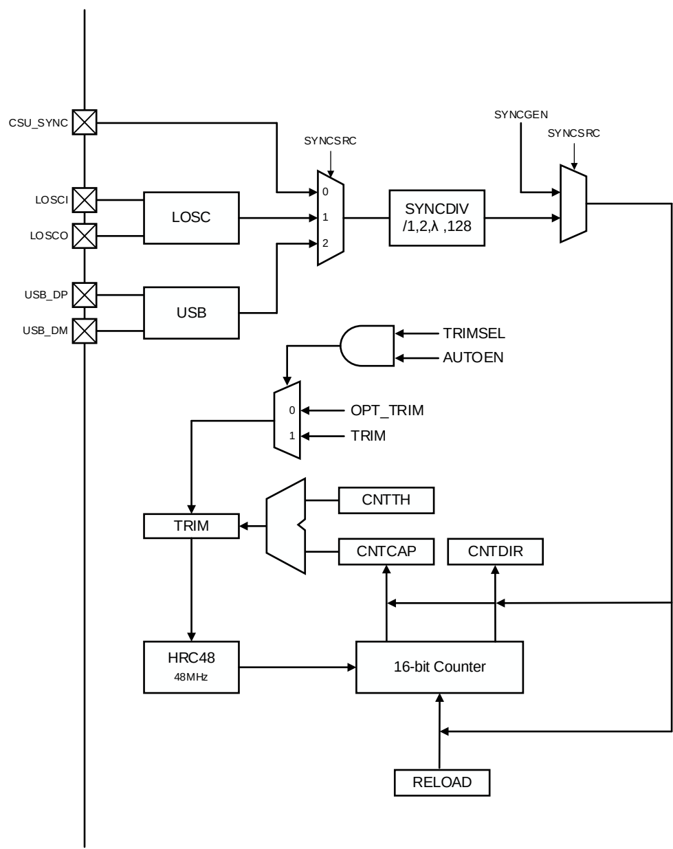
图 11-1 CSU 结构图
