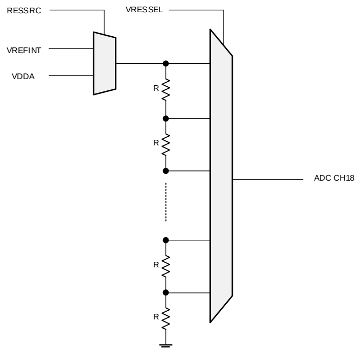
图 16-25 V_{RES} 分压
