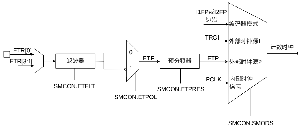
图 20-5 外部触发输入模块
