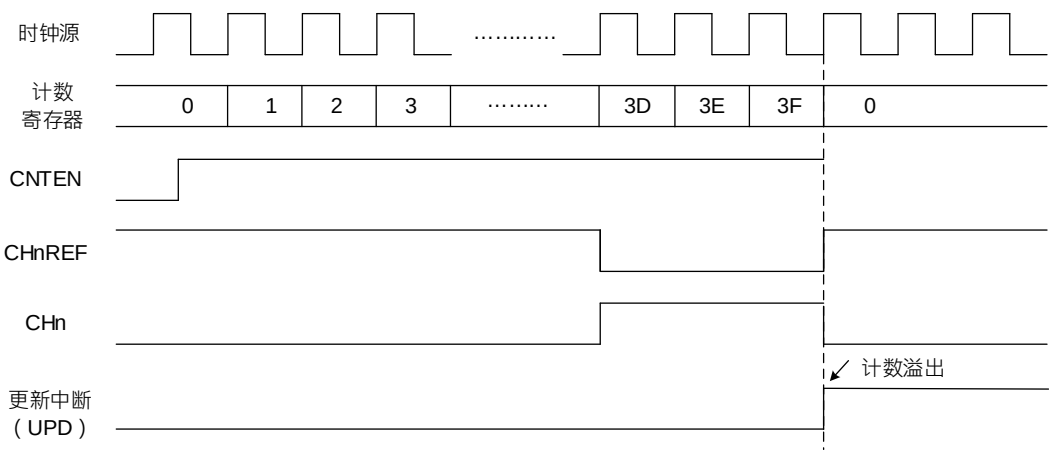
图 21-16 单脉冲模式
