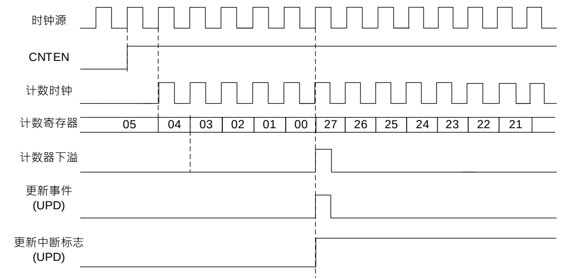
图 19-10 计数器递减计数时序图
