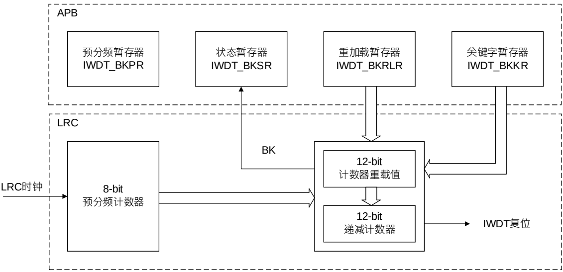
图 23-1IWDWT 架构图
