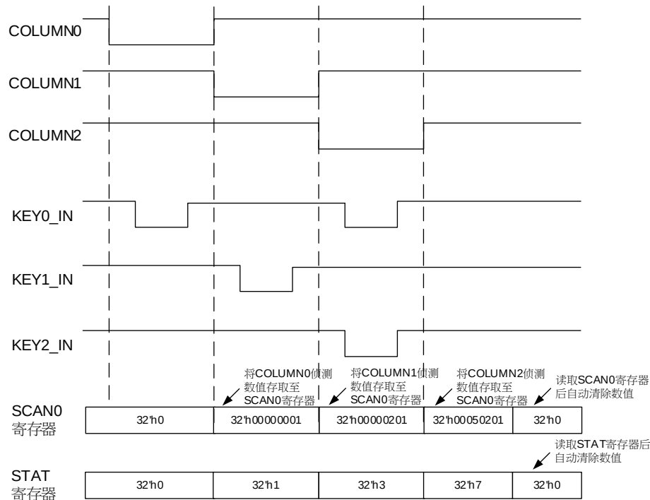
图 12-10 KBCU 按键扫描
