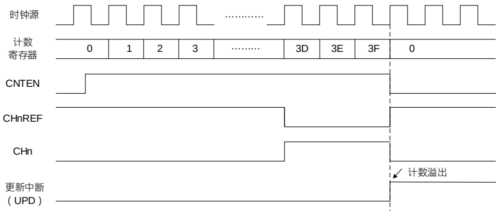
图 19-21 单脉冲模式
