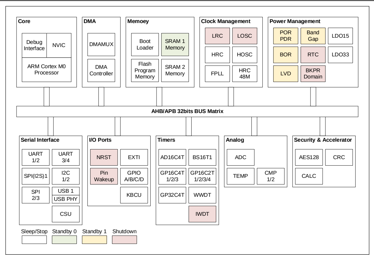
图 1-1FS026x7L 系统框图
