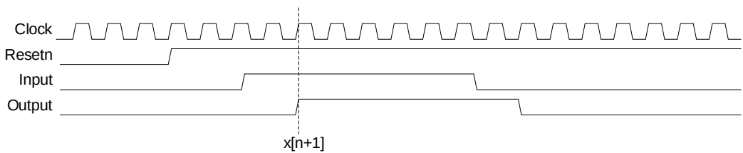
图 14-5 防抖动输出
