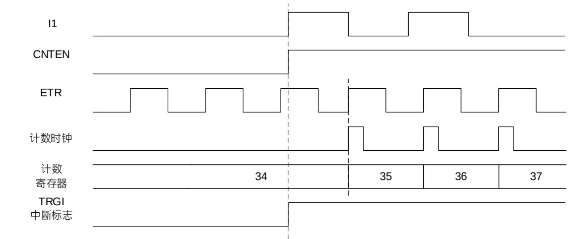
图 19-27 外部时钟源 2+触发模式下的控制电路
