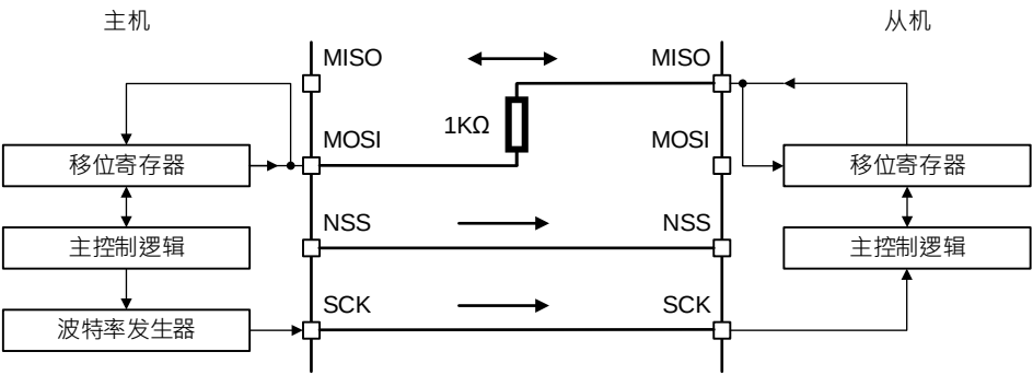
图 27-4 半双工通信
