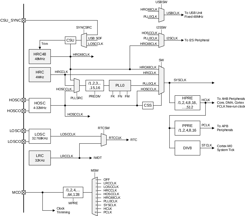
图 4-2 时钟架构图
