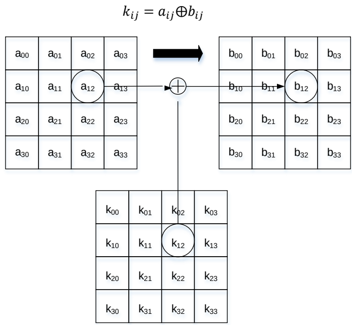
图 9-1 轮密钥加
