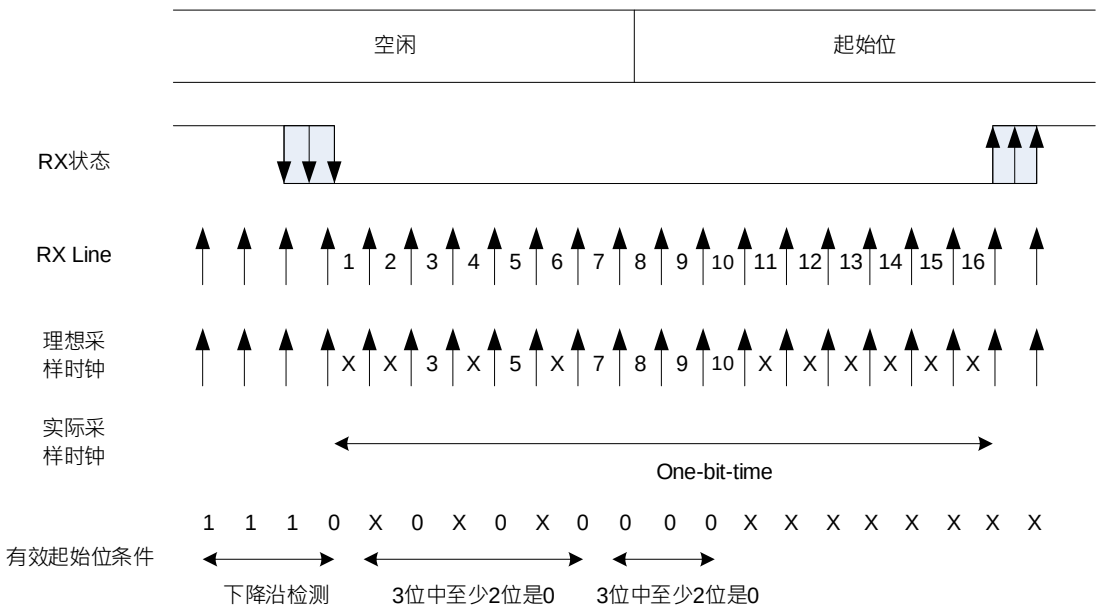
图 14-6 起始位侦测
