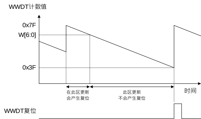
图 24-3WWDT 时序图
