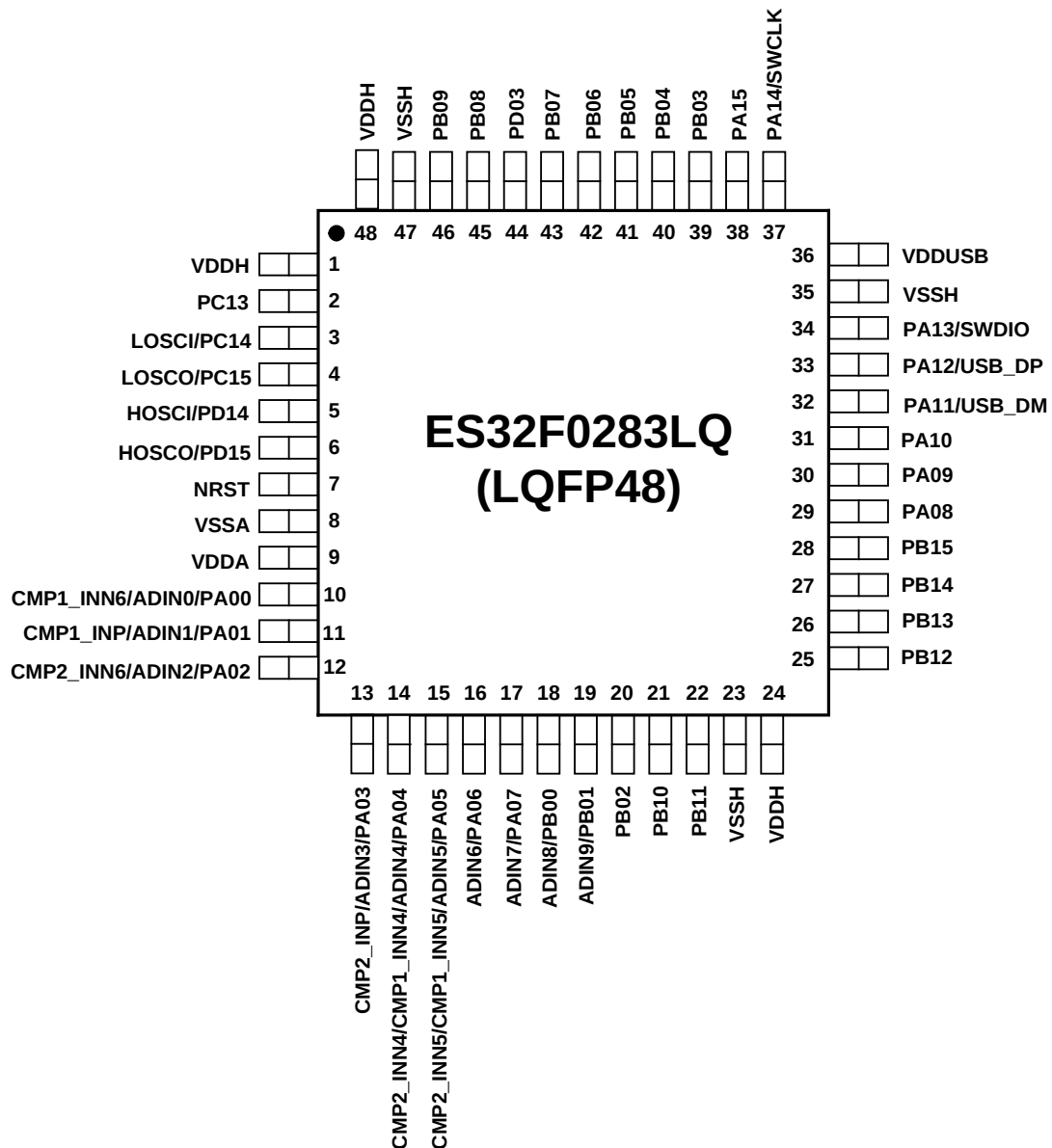
图 3-3 ES32F0283LQ 48-Pin (7x7mm) LQFP 引脚图
