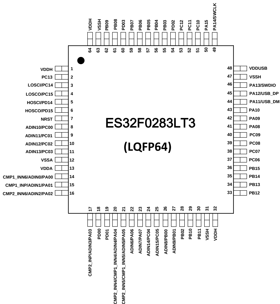
图 3-1 ES32F0283LT3 64-Pin (10x10mm) LQFP 引脚图
