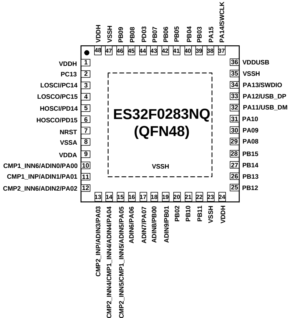
图 3-4 ES32F0283NQ 48-Pin (5x5mm) QFN 引脚图
