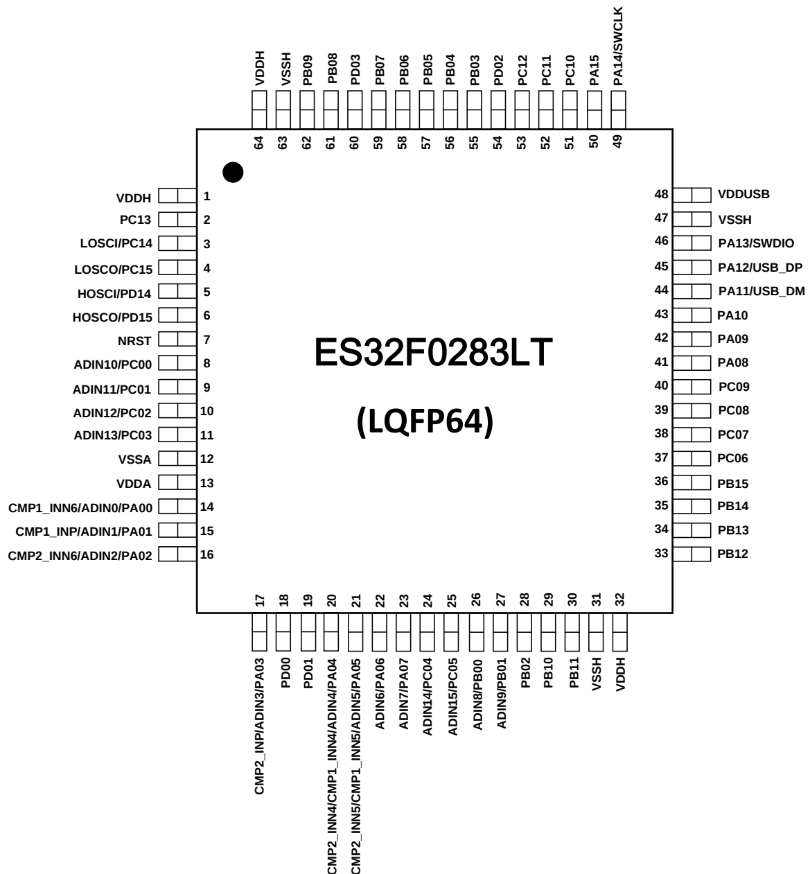
图 3-2 ES32F0283LT 64-Pin (7x7mm) LQFP 引脚图
