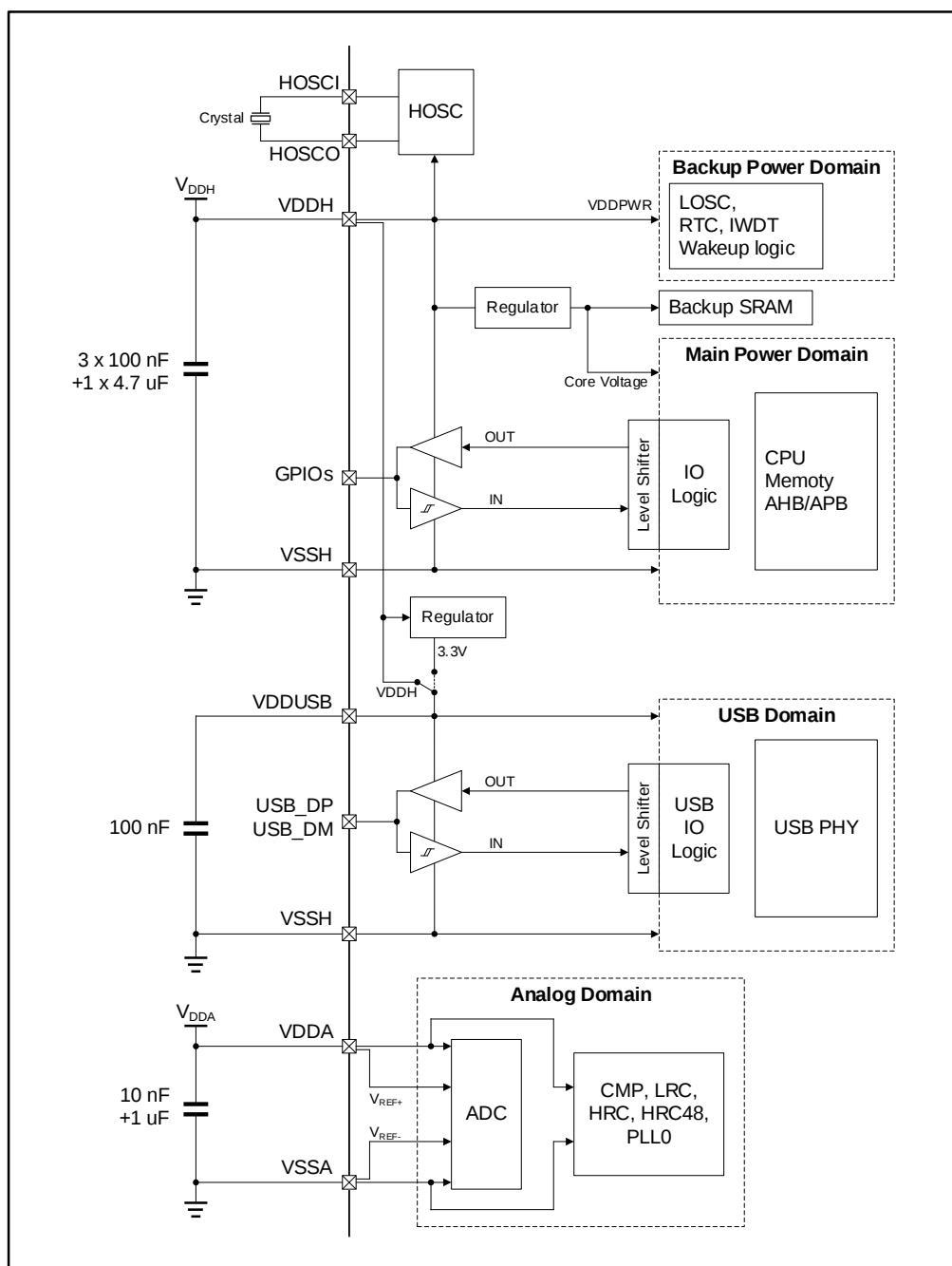
图 5-1 芯片电源
