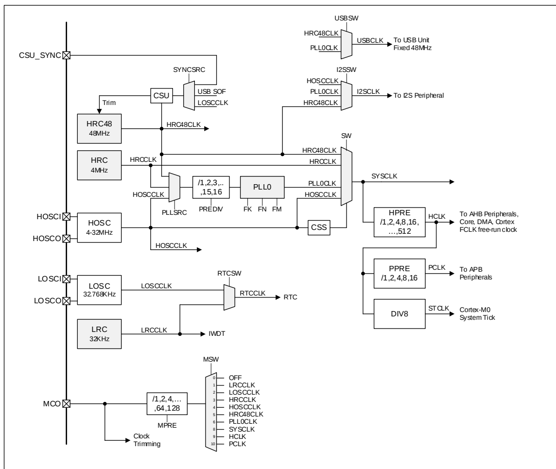
图 2-2 系统时钟树
