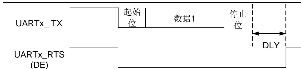
图 22-14 驱动开启, AADINV=0
