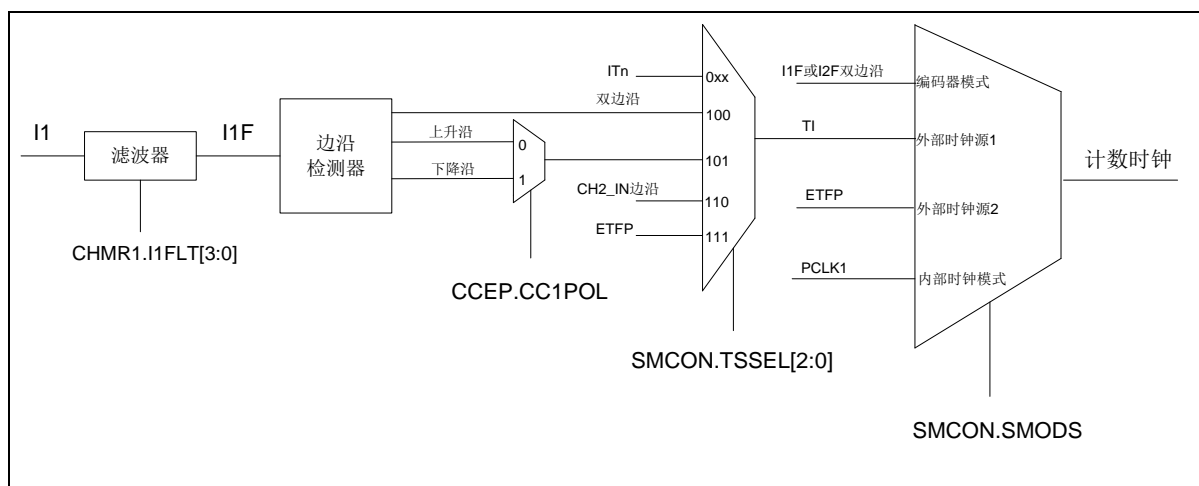
图 17-4 I1 外部时钟连接
