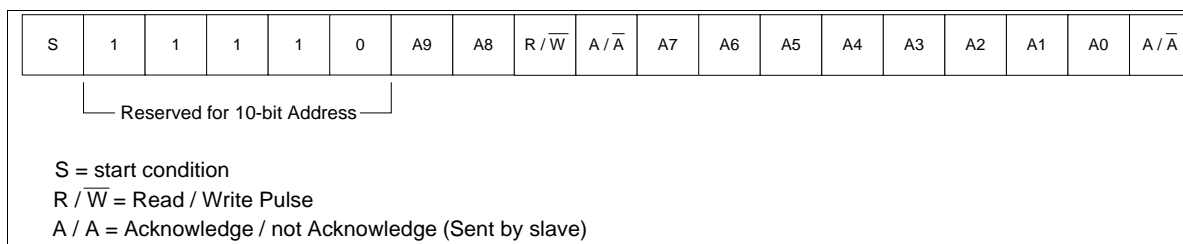
图 20-5 10 位地址格式
