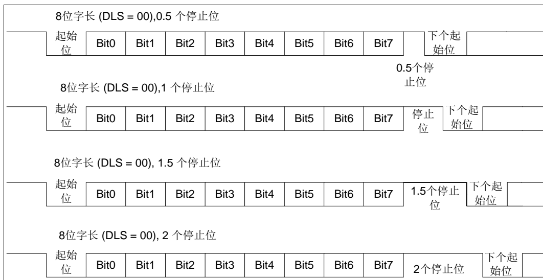
图 22-3 停止位配置
