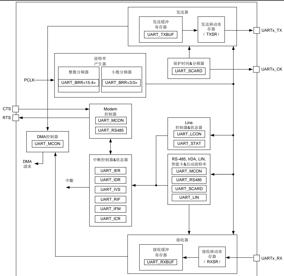
图 22-1 UART 框图
