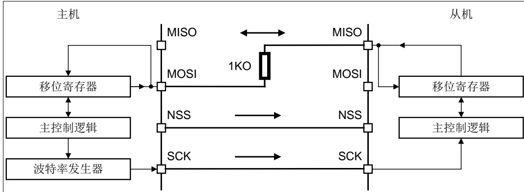
图 21-4 半双工通信
