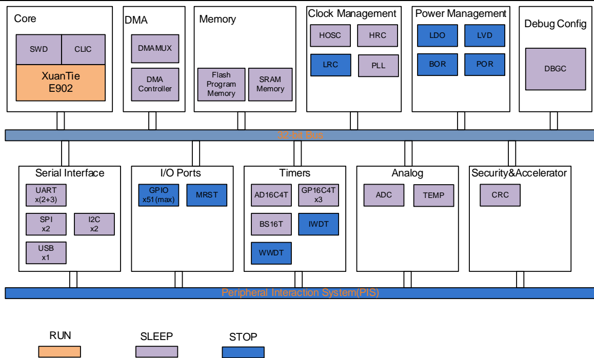
图 2-1 系统框图
