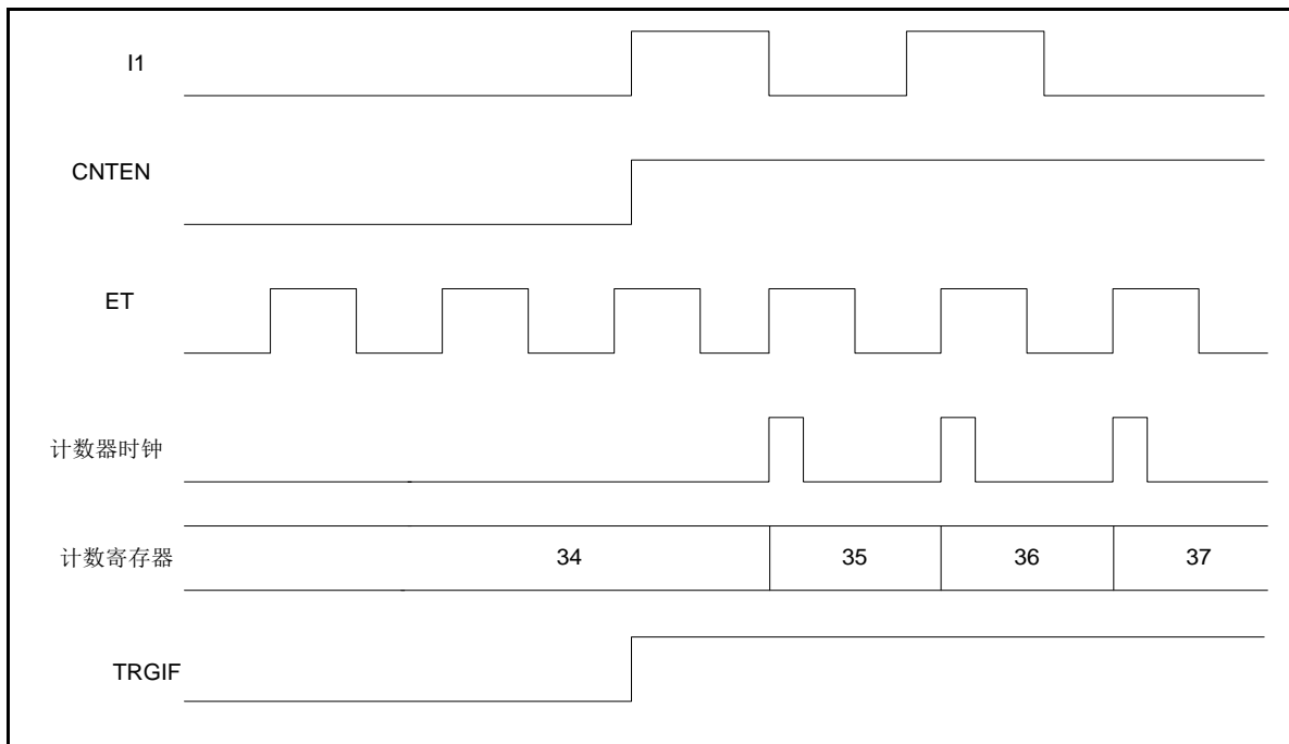
图 18-24 外部时钟源 2+触发模式下的控制电路
