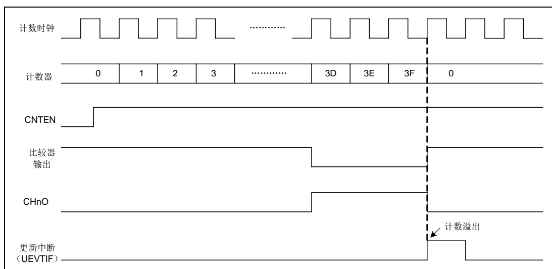
图 17-18 单脉冲模式
