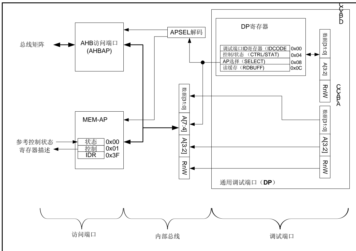
图 25-2 MEM-AP 地址映射
