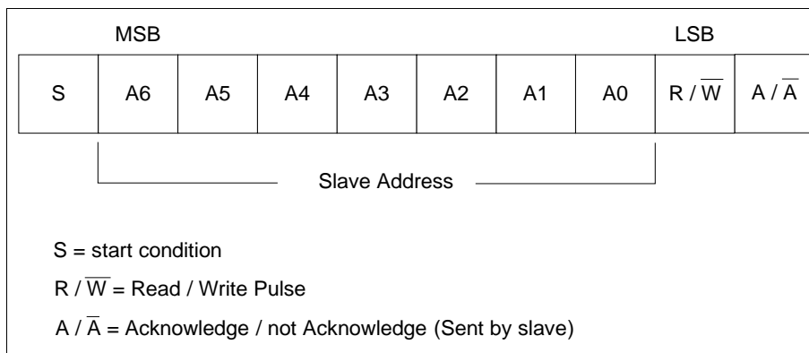
图 20-4 7 位地址格式
