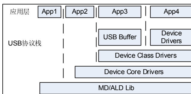
图 3-3 USB 协议栈设备驱动结构
