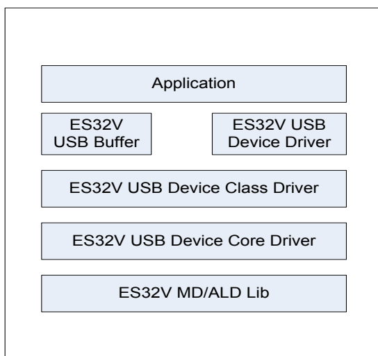
图 3-1 USB 协议栈设备驱动结构
