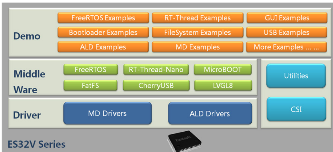
图 1-1 ES32V SDK 框架
