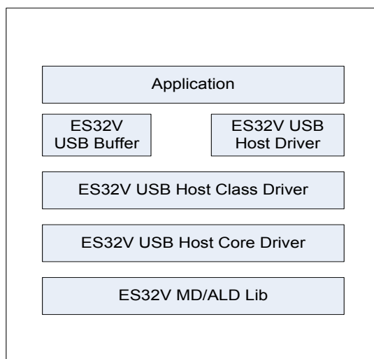
图 3-2 USB 协议栈主机驱动结构
