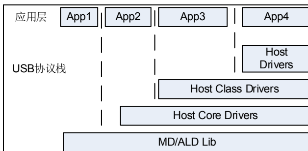
图 3-4 USB 协议栈主机驱动结构
